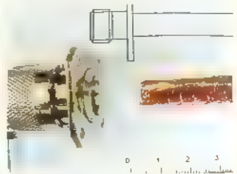
Opsluiten van de ruimte om de kern met teflon-tape. Het chassisdeel is voorbereid om straks gemakkelijk te kunnen solderen
